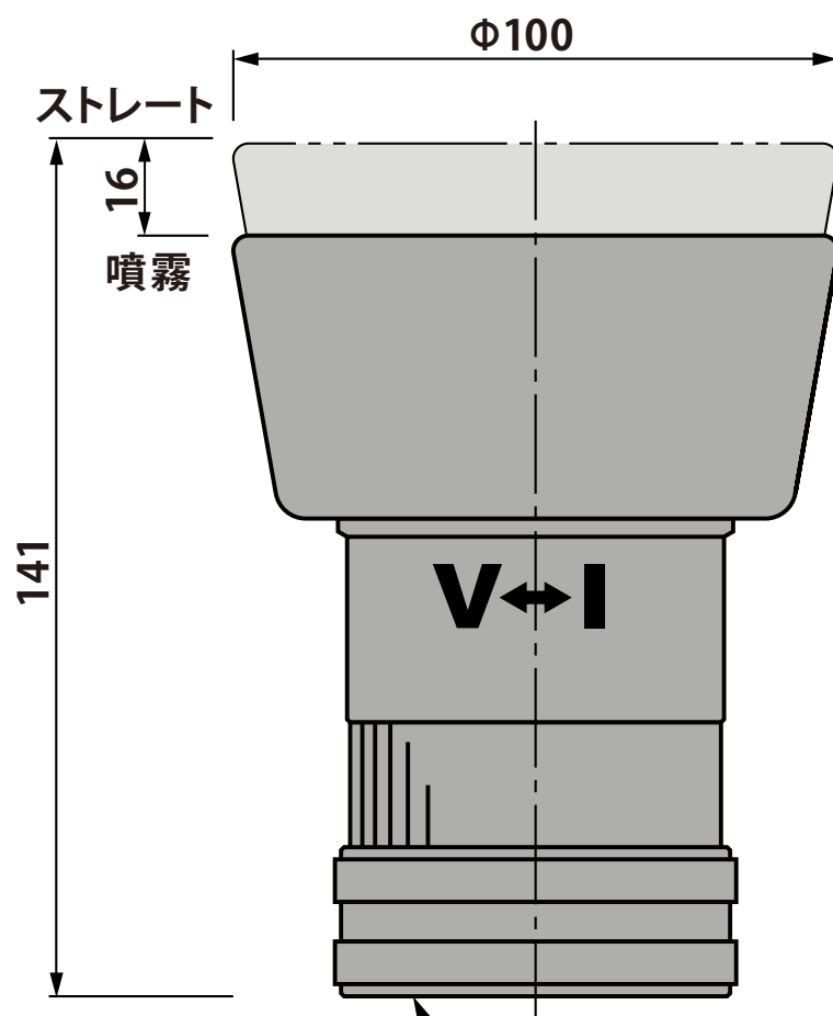
呼び65 消防用ノズルチップ雌結合金具 Φ55 10山/25.4
